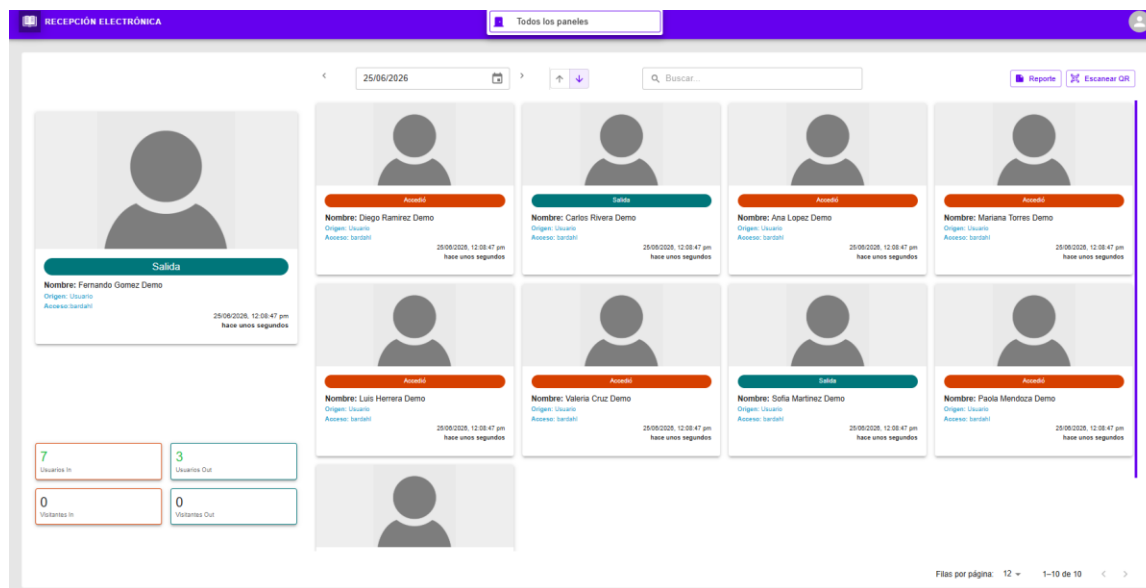
Ilustración 16. Kiosco
