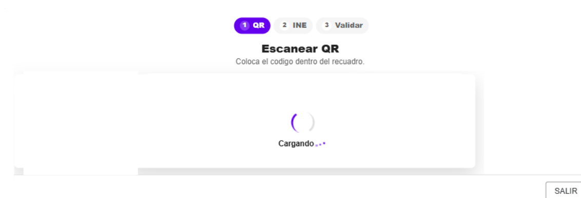
Ilustración 17. Escáner QR
