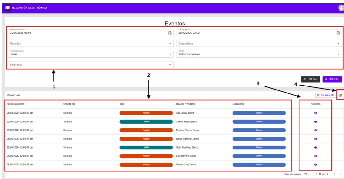
Ilustración 18. Eventos
