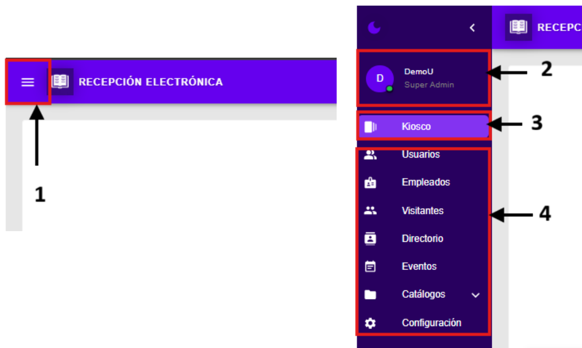
Ilustración 7. Menú principal
